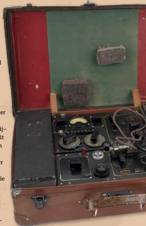
Spionagezender van het koffertype B2, zoals destijds werd gebruikt door geheim agenten die boven bezet gebied waren gedropt.
