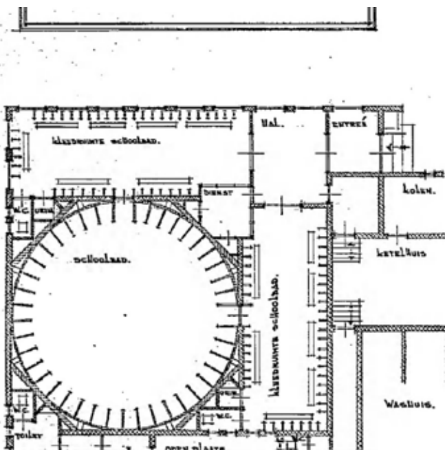
Plattegrond van het schoolbad: Boven en rechts omkleedruimtes voor de jongens en de meisjes. Midden: alle doucheplekken in een cirkel
